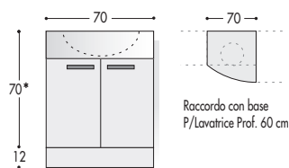
BASE RACCORDO A TERRA: H. 70+12 (escluso top)
